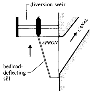
(d) Intake with bedload-diverting sill
