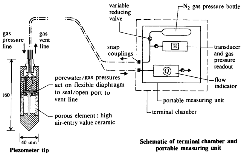
Fig. 7.3 Pneumatic piezometer
